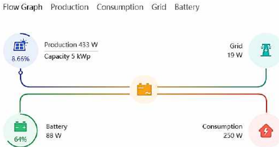
Рисунок 1 – Приклад системи моніторингу роботи гібридної СЕС потужністю 5 кВт
