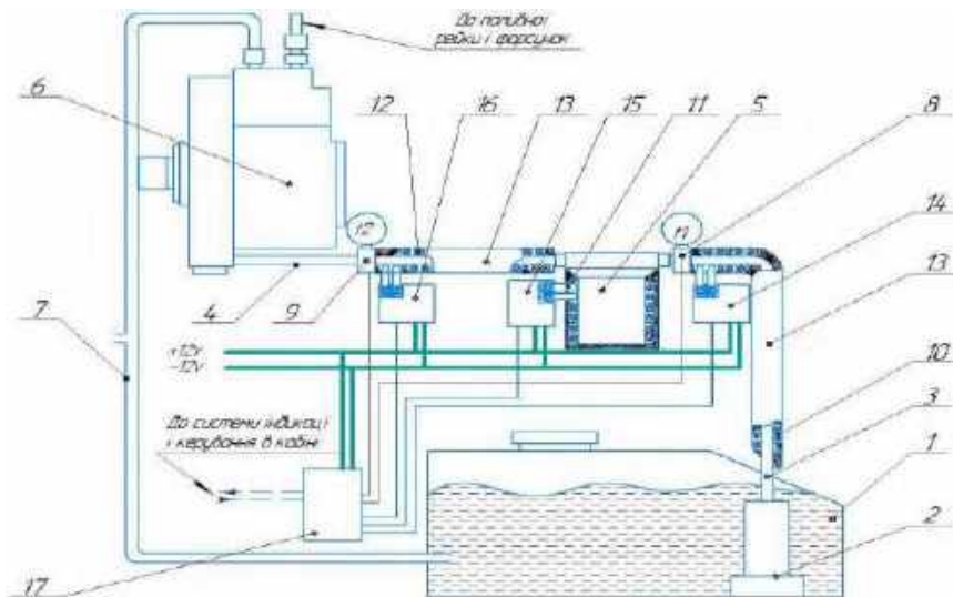
Рис. 1. Система підігріву пального для дизельних двигунів:
