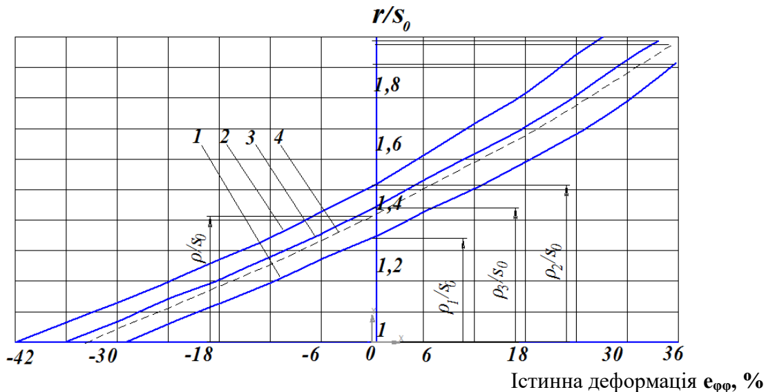
Рис. 3. Розподіл тангенціальних деформацій \epsilon_{\phi} за товщиною полоси при профілюванні (1, 2, 3) і чистому круговому вигині (4) за умови \frac{r_z}{s_0} = 1 та \alpha = \pi/2 ; 1 – на осі симетрії місця вигину ( x_0 = 0,5b_{\text{виг}} ); 2 – на межах місця вигину та плоских елементів ( x_0 = 0,5b_{\text{виг}} \pm 0,5b_{\text{виг}} ); 3 – в перерізах з потоншенням \Delta s = 0,5\Delta s_{\text{max}} ( x_0 = 0,5b_{\text{виг}} \pm 0,182b_{\text{виг}} )
