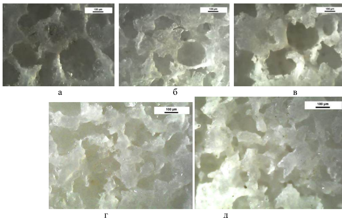
Рис. 2. Порова структура ПТФЕ сформована різними пороутворювачами: а – 100C; б – 75C25N; в – 50C50N; г – 25C75N; д – 100N
