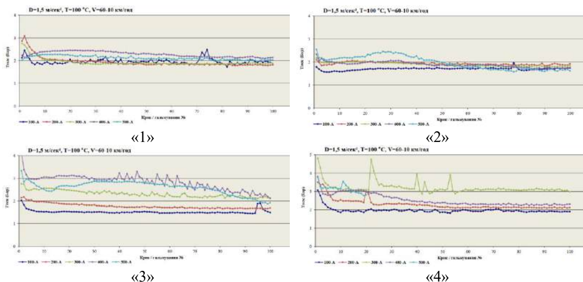
Рис. 5. Результати зносних гальмувань на швидкості 10-60 км/год Джерело: складено автором на основі протоколів випробувань
