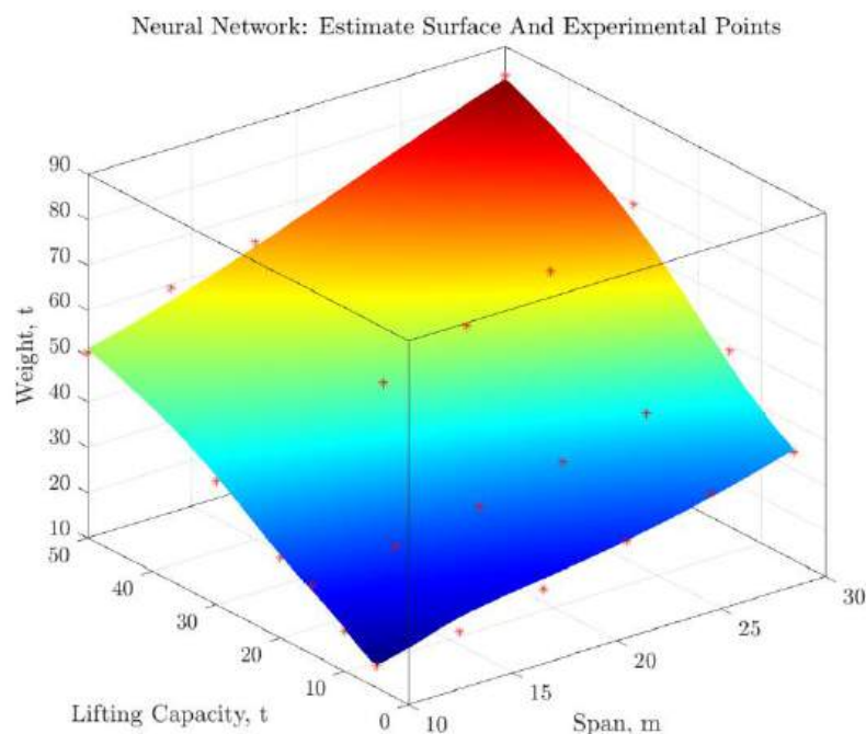
Рис. 7. Результат розрахунку маси крану в залежності від прольоту і вантажопідйомності за допомогою нейромережі для кранів режимів роботи А6-А8
