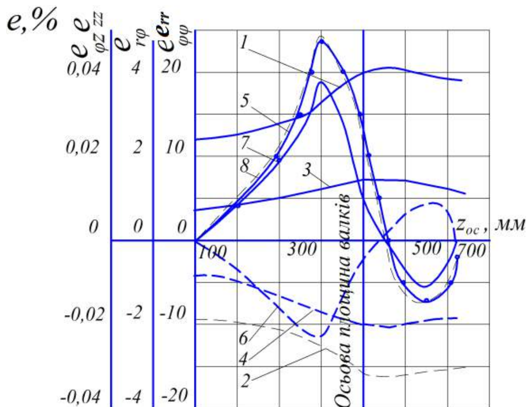
Рис. 2. Графіки зміни компонентів тензора деформацій e_{\phi\phi} (1, 2), e_{\rho\phi} (3, 4), e_{\phi z} (5, 6) і e_{zr} (7, 8) металу місця вигину швелера 150 \times 100 \times 2 мм уздовж ділянки плавного переходу в третій формувальній клітці ( 30 - 50^\circ ) на зовнішній (1, 2, 5, 7) і внутрішній (2, 4, 6, 8) поверхнях
