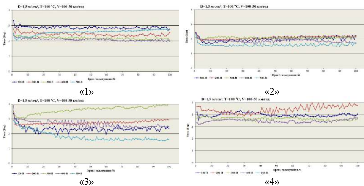
Рис. 6. Результати зносних гальмувань на швидкості 10-60 км/год Джерело: складено автором на основі протоколів випробувань
