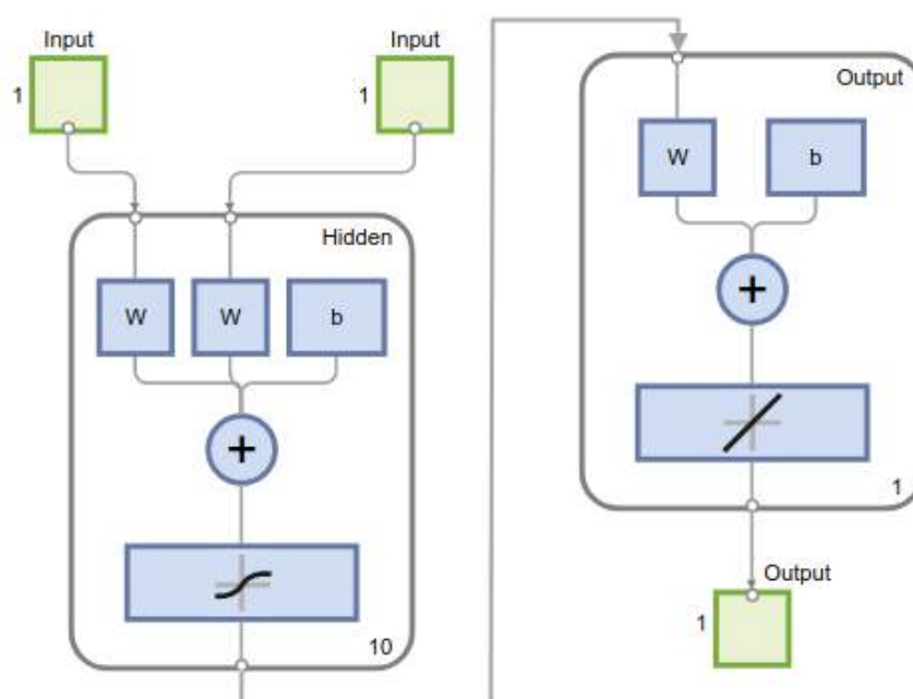
Рис. 4. Структура нейронної мережі для розрахунку ваги мостових кранів
