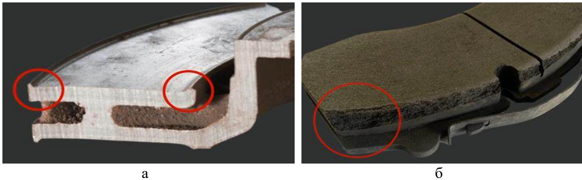
Рис. 1. Зношування гальмівної колодки та диска: а) борозди на диску; б) руйнування країв гальмівної колодки
