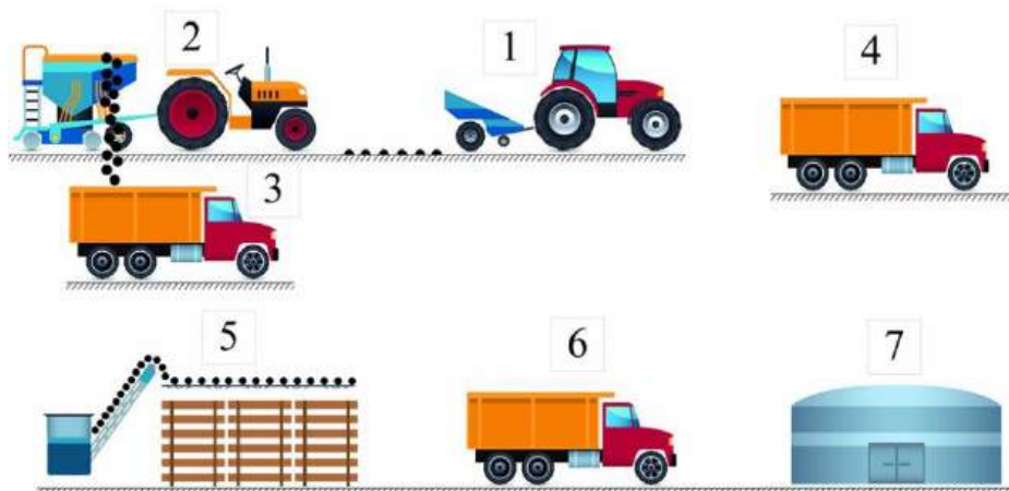
Рис. 2. Схема збирального процесу картоплі двофазним способом: 1 – картоплекопувач; 2 – комбайн підбирач; 3 – супроводжуючий автомобіль; 4 – завантажений автомобіль; 5 – сортувальний пункт; 6 – завантажений автомобіль; 7 – сховище.
