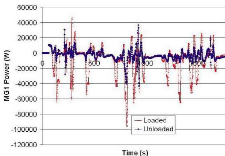
Рис. 2. Результати моделювання ICEHV: потужність першого мотор-генератора з багаторежимною конфігурацією силової установки на трасі "Місто-передмістя"
