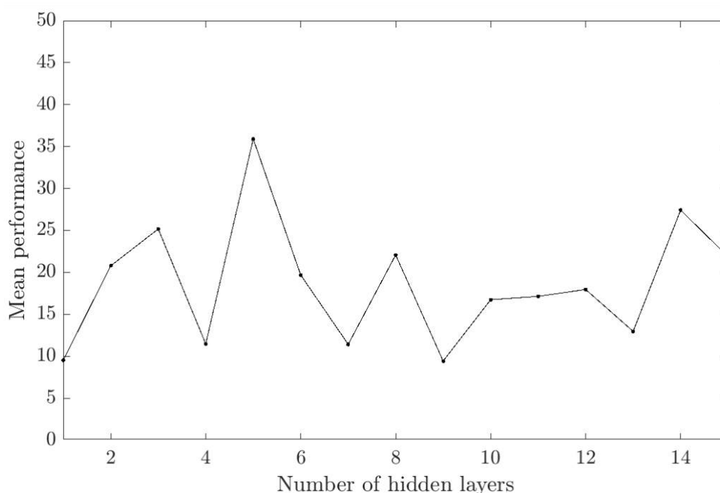
Рис. 3. Залежність середньої точності від кількості прихованих шарів
