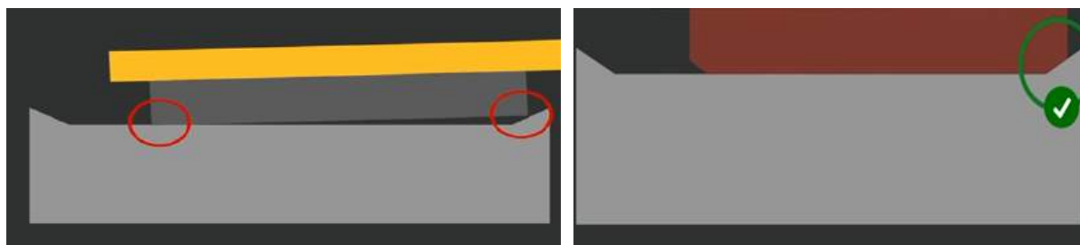
Рис. 3. Контакт нової удосконаленої колодки та зношеного диска: а) контакт традиційної колодки та зношеного диска б) контакт удосконаленої колодки та зношеного диска
