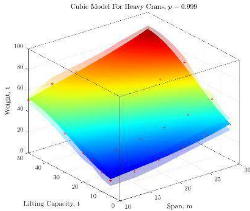
Рис. 2. Результат розрахунку маси крану в залежності від прольоту і вантажопідйомності на основі отриманої функціональної залежності для кранів режимів роботи: А6-А8
