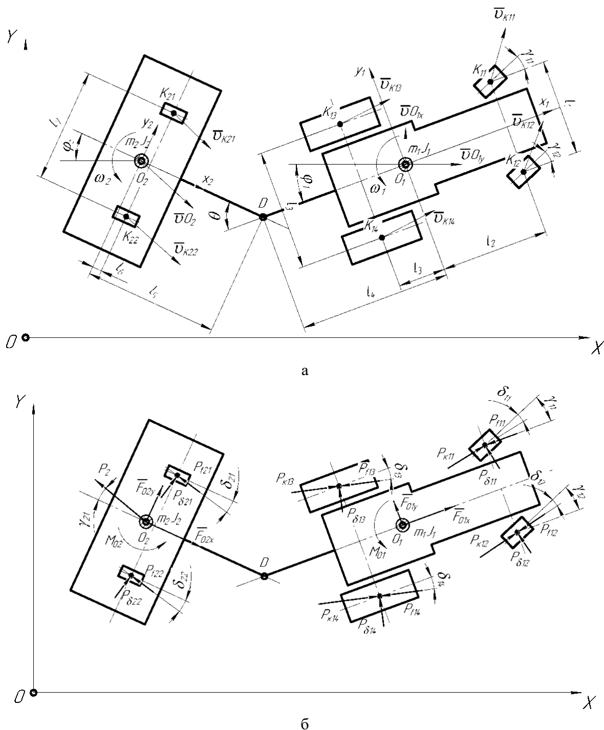
Рис. 1. Кінематична (а) та динамічна (б) моделі плоско-паралельного руху двохелементного (двох масового) посівного машинно-тракторного агрегату
