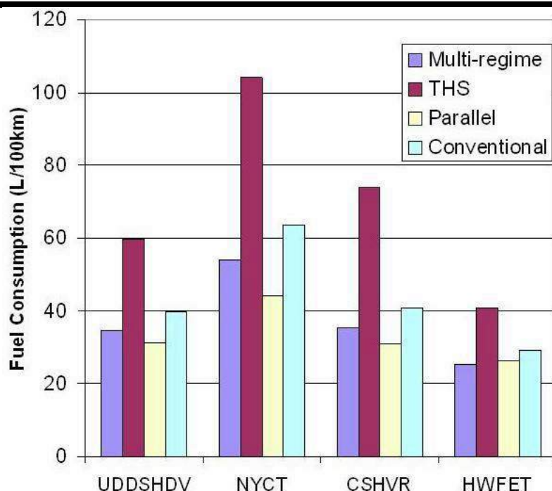
Рис. 1. Результати моделювання ICEHV: витрата палива у завантаженому автомобілі
