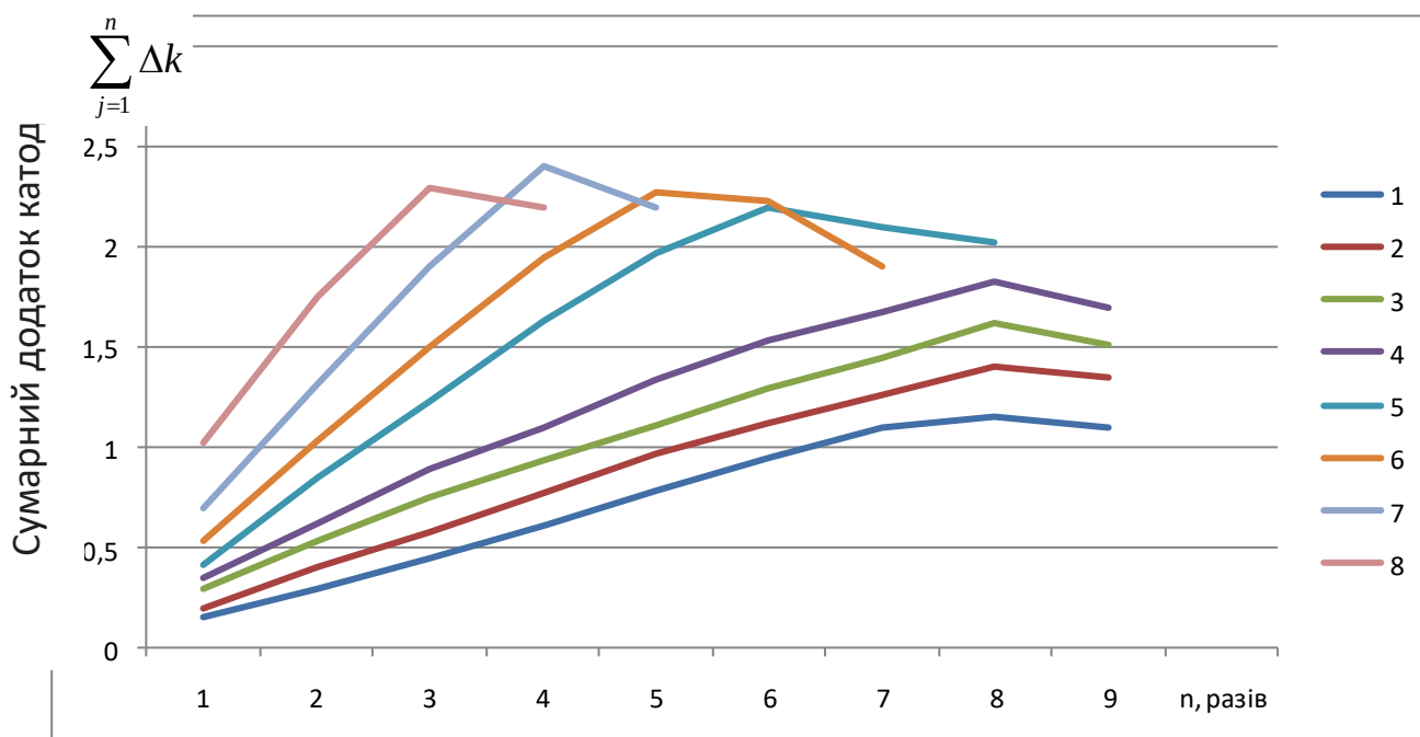
Рисунок 2. Залежність додатку ваги катода - \sum_{j=1}^n \Delta k при ЕІО від кількості
