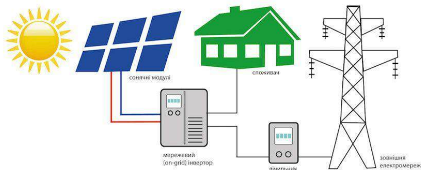
Рис. 3. Загальна схема гібридної сонячної електростанції.
