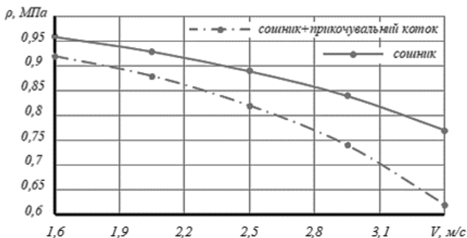
Рис. 3. Залежність твердості ґрунту \rho у посівній борозні від швидкості руху сіялки V
