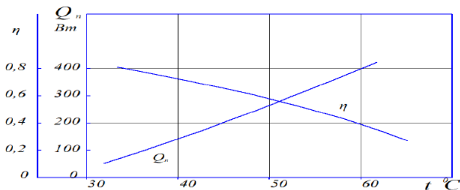
Рис. 2 – КПД та інтегральні теплові втрати геліоводонагрівача в залежності від температури t геліоприймача
