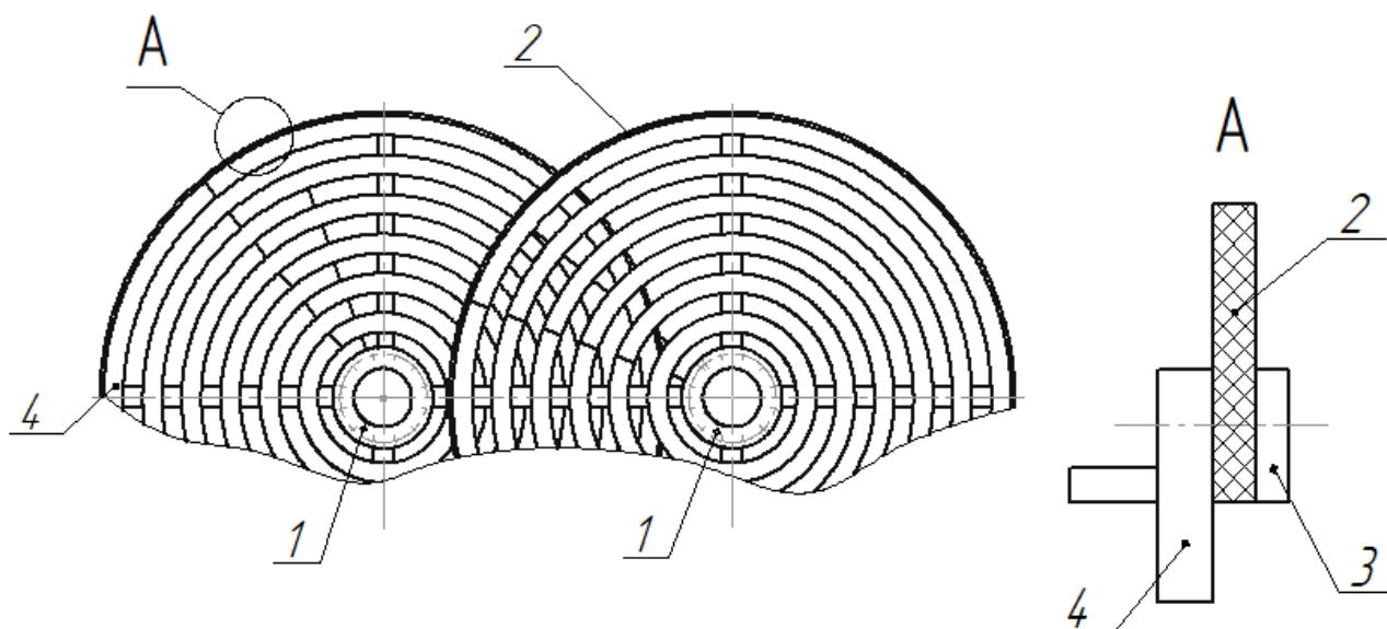
Рис. 1. Модернізований транспортуєчий шнек дифузійного апарату
