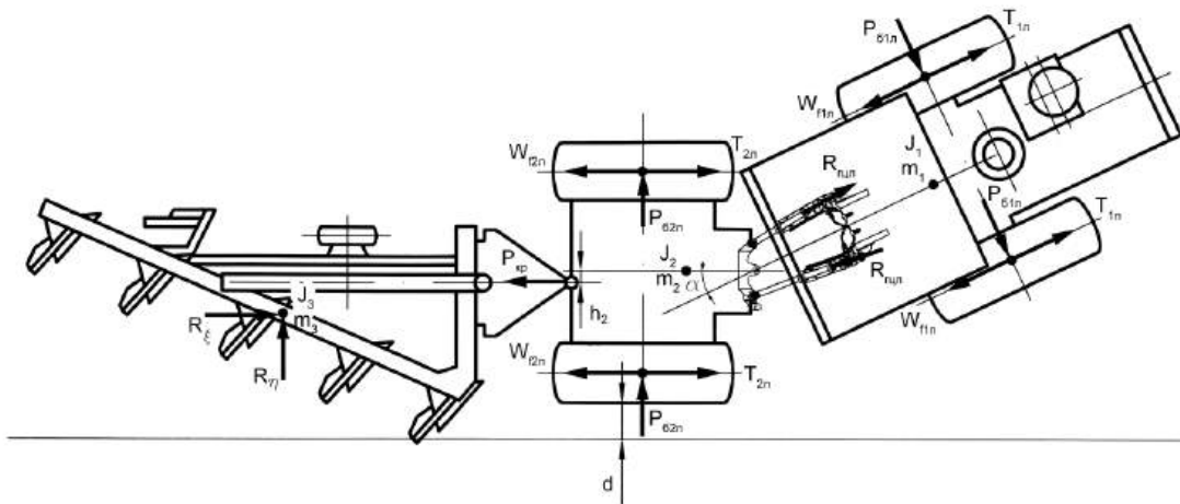
Рис. 1 – Схема дії сил на колесах трактора при орних роботах
