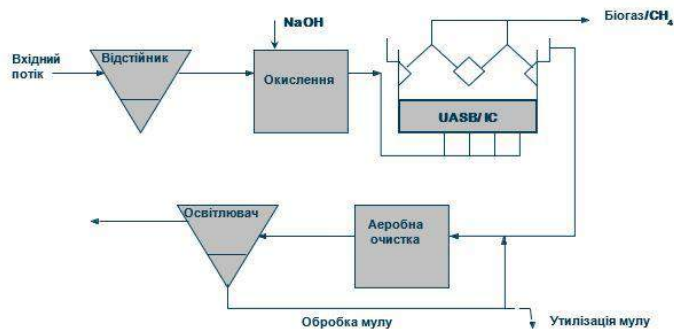
Рис. 1 Схема технологічного процесу очищення стічних вод
