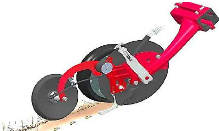
Рис. 4. Секція з монодиском
