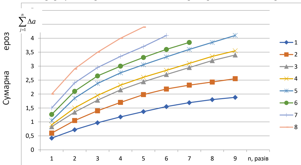
Рисунок 1. Залежність сумарної ерозії аноду - \sum_{j=1}^n \Delta a при ЕІО від кількості
