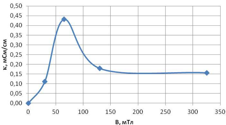
Рис. Залежність зміни питомої електропровідності розчину солей від магнітної індукції при швидкості руху розчину 0,4 м/с
