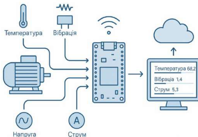
Рис. 1. IoT–система для дистанційного моніторингу та раннього виявлення несправностей електродвигуна
