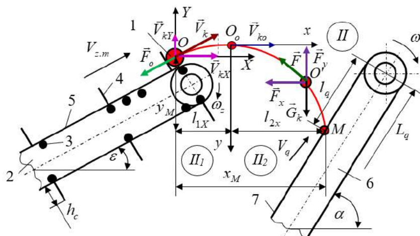
Рис. 1. Схема до розрахунку дальності польоту компонента вороху:
