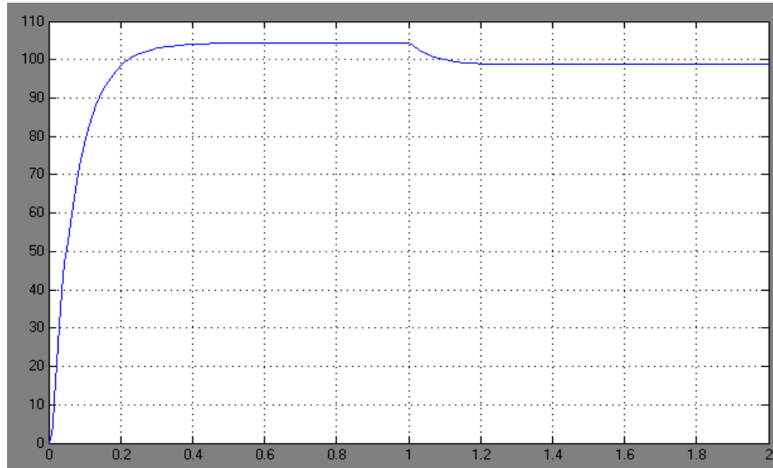
Рис. 2. Графік швидкості перехідного процесу \tau_{pp}=0,2\text{с} .
