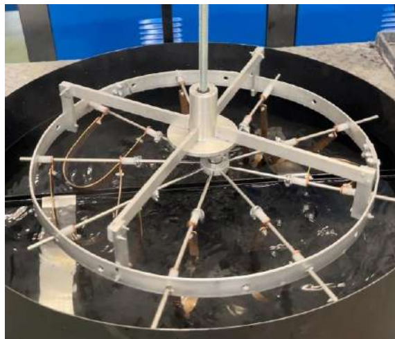
Рис.1. Загальний вигляд теплового двигуна з робочими елементами – функціональним сплавом Camital
