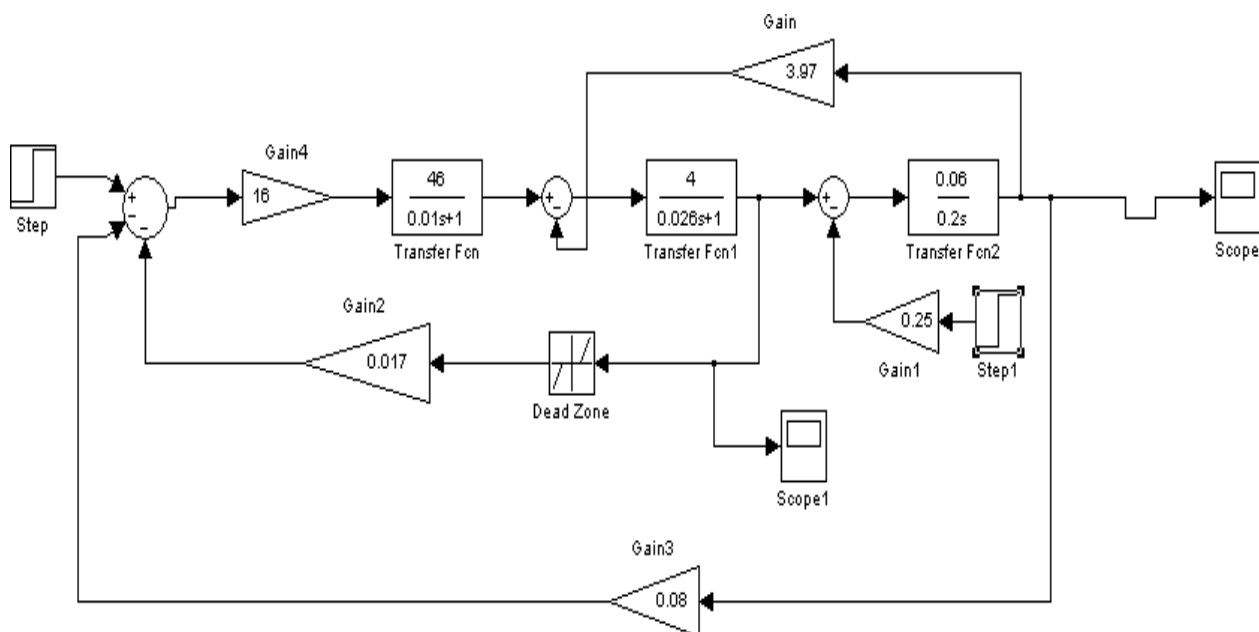
Рис.1. Імітаційна модель управління зворотним зв'язком у середовищі моделювання MatLab/Simulink.
