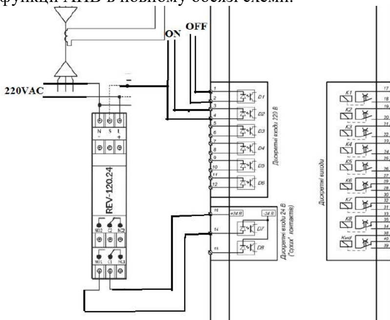
Рис.1. Фрагмент удосконалення схеми підключення дискретних входів пристрою РЗЛ–05М
