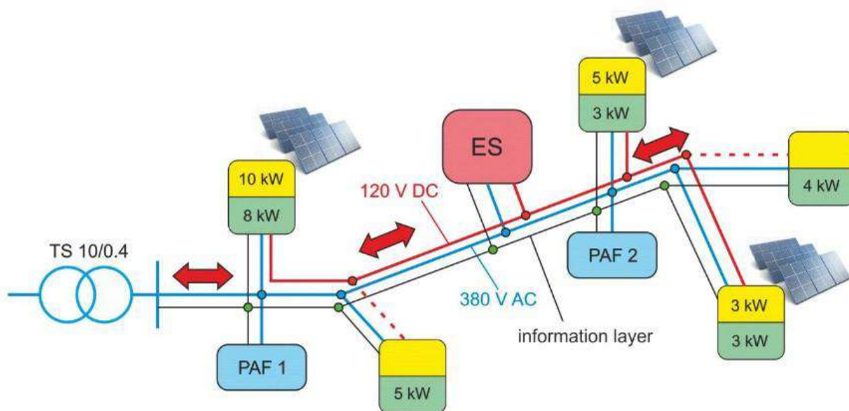
Рис.1. Структурна схема локальної Smart Grid [2]
