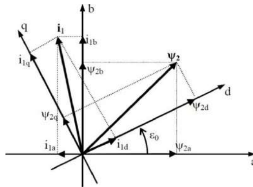
Рис. .1 – Розташування векторів АД
