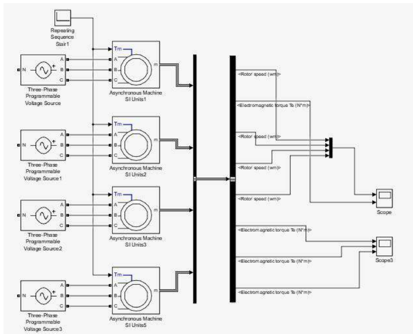
Рис.1. Модернізована віртуальна модель для дослідження асинхронного електродвигуна подачі сировини в установку для подрібнення кормів.
