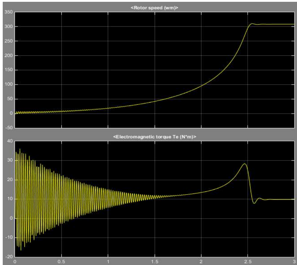
Рис.2. Перехідний процес зміни швидкості та моменту при підключенні до електродвигуна з навантаженням ( M=9,5 Нм) та частоти f=50 Гц.
